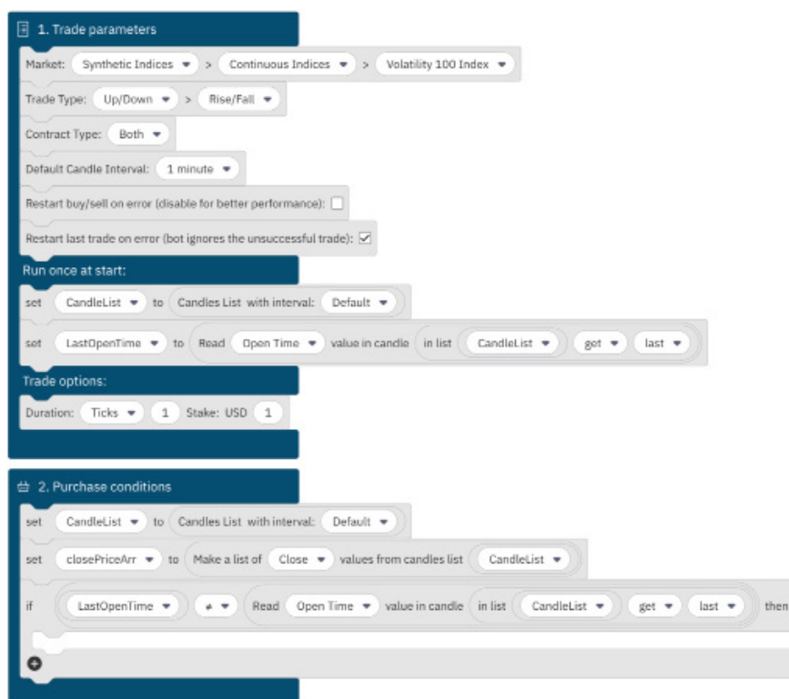
Figure 26. Deriv Bot
